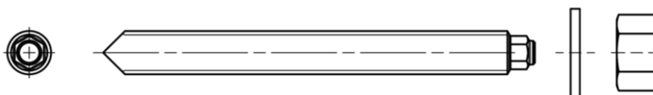
Figure 3 : Tiges métalliques – tige filetée ; 6 mm ≤ d ≤ 30 mm
